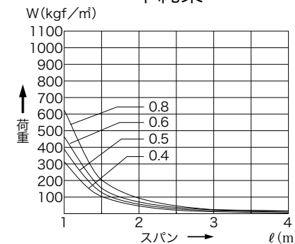
単純梁
