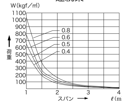
連続梁
