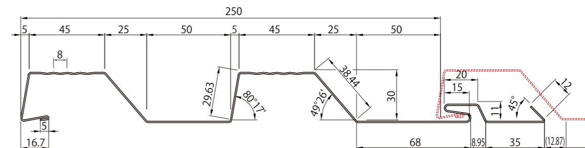
【250K型スパンドレル】
